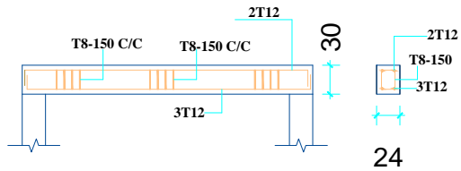
BEAM - B : 24x30
